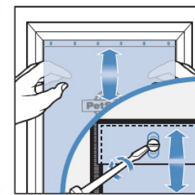
FIG.9 Ajuste vertical Movimente a aba para cima ou para baixo para ajustá-la na posição. Quando estiver bem, aperte os parafusos.
