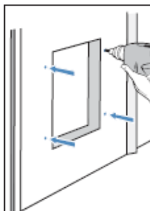
FIG.5 Retire a moldura e com o berbequim usando a broca de 7mm (1/4"), faça os buracos, conforme indicado.
