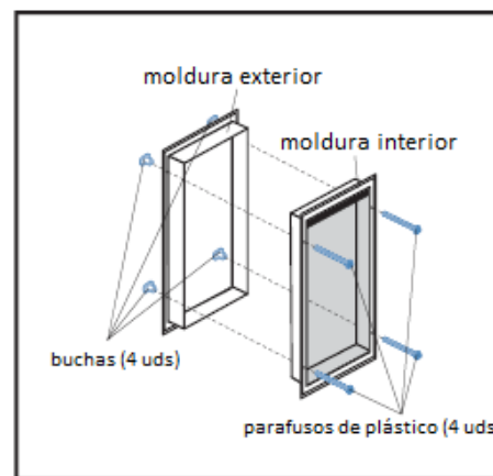
FIG.6 Encaixe a moldura exterior no recorte e coloque as buchas através dos orifícios na moldura e na porta. Coloque a moldura interior no recorte. Aperte os parafusos de plástico através dos orifícios na moldura (não aperte demasiado). Corte o excesso dos parafusos de plástico, com cuidado para não danificar a moldura externa. Retire, se necessário.
